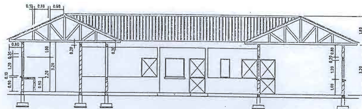
COUPE A-A
